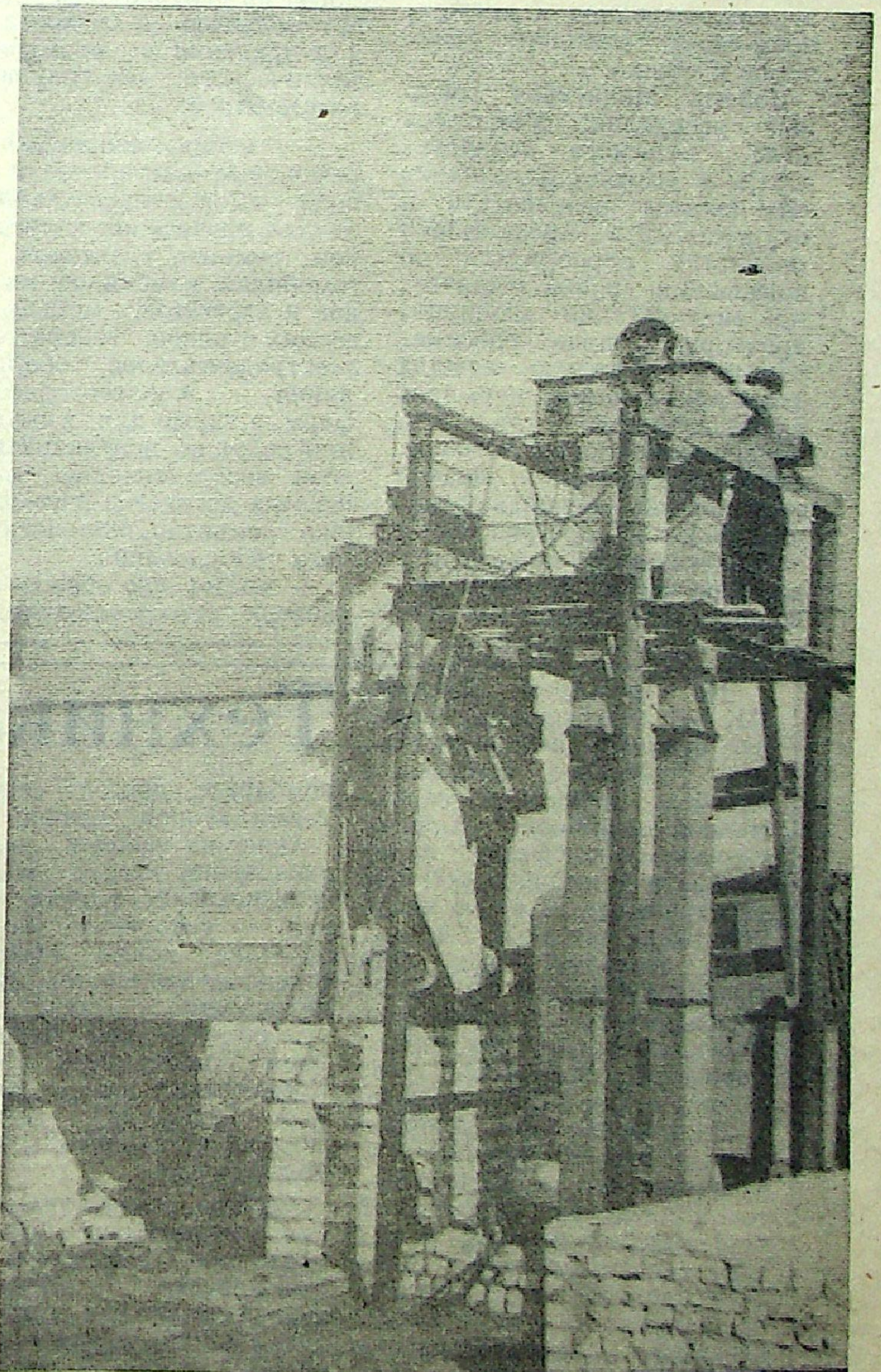
На четвертом отделении совхоза «Мирный» завершаются монтажные работы зерноочистительного агрегата ЗАП-50. Его производительность — 50 тонн зерна в час.
